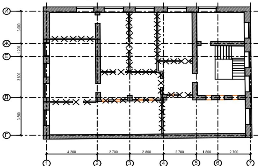
План демонтажных работ 2-го этажа (3-й этап)
